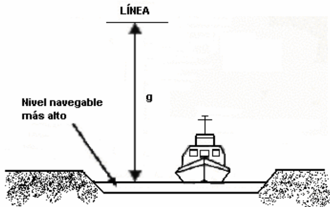
Figura 8 (b). Distancia “g” en cruces con ríos, cauces de agua, canales navegables
