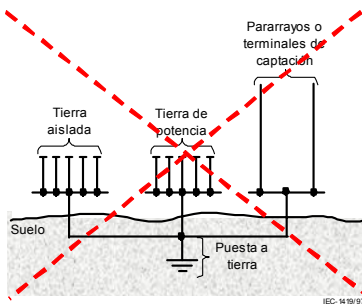
Figura 11. Una sola puesta a tierra para todas las necesidades (prohibido).
