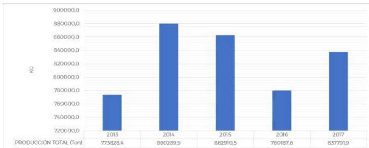
Gráfico 3. Producción anual de barras corrugadas de baja aleación.
