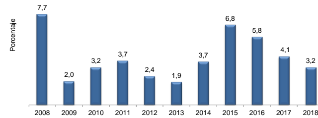
Desempleo (%)
