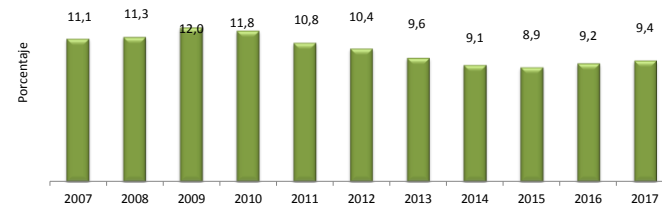
Desempleo (%)
